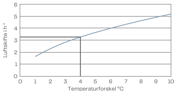
Beregne luftskifter ved termisk opdrift
