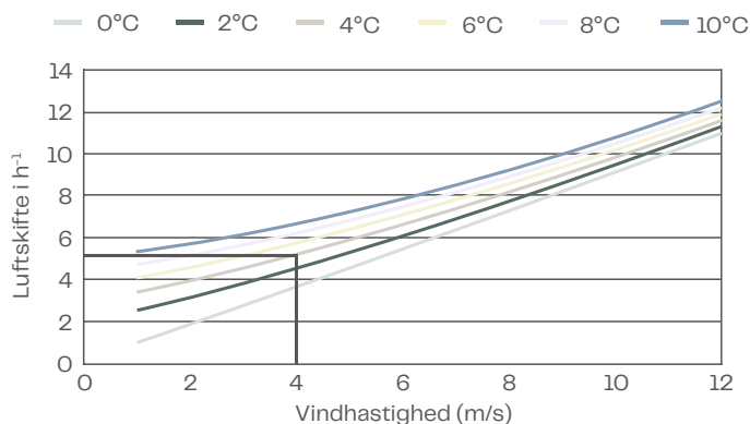
Beregne luftskifter ved termisk opdrift og vind
